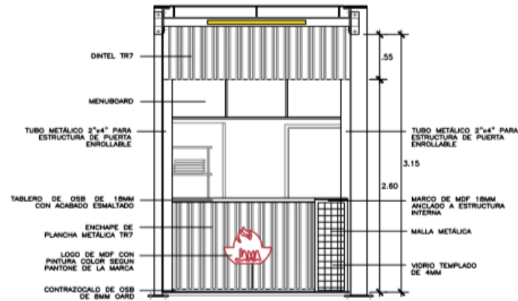
FACHADA ESCALA 1/50
