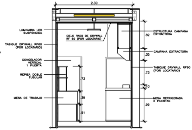
CORTE E-E ESCALA 1/50
