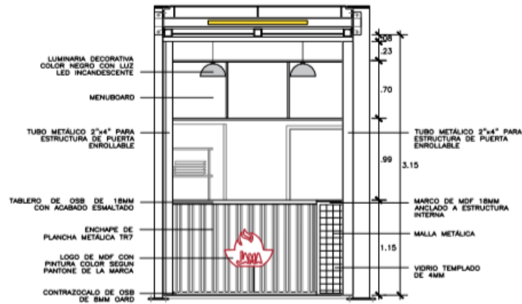
ELEVACION FRONTAL ESCALA 1/50
